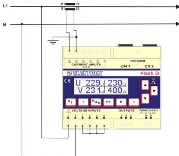
Bassa tensione Fase Neutro 1 TA Configurazione 1Ph/2W
